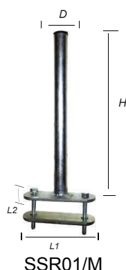
SSR01/M
