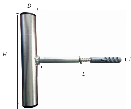
SSR01/M
